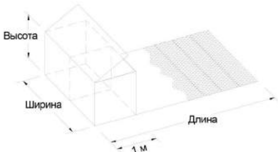
Рисунок 2. Конструктивная схема габрионной конструкции коробчатой с армирующей панелью.
